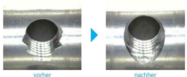
Außermittige Querbohrung (Aluminium)
