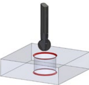
PLANE BOHRUNG
