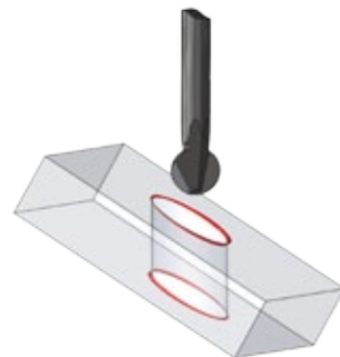
GENEIGTE OBERFLÄCHENBOHRUNG
