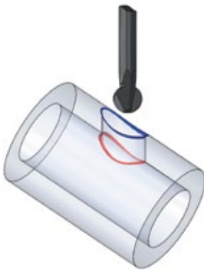
GENEIGTE QUERBOHRUNG
